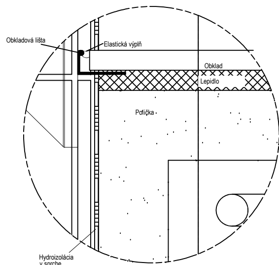
DETAIL UKONČENIE POLIČKY
