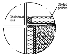
DETAIL UKONČENIE POLIČKY
