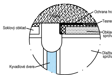
DETAIL NAPOJENIE SPRCHOVÝCH DVERÍ
